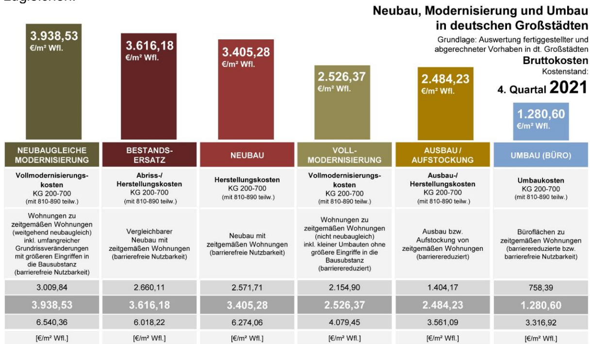
Abbildung 22: Baukosten-Vergleich realisierter Wohnungsbauvorhaben aus den Bereichen: (1.) Neubaugleiche Modernisierung mit Um- und Anbau von Wohngebäuden der 1950er und 1960er Baujahre zu zeitgemäßen Wohnungen, (2.) Bestandsersatz von Wohngebäuden, (3.) Neubau von Wohngebäuden, (3.) Vollmodernisierung von Wohngebäuden, (4.) Ausbau von Dachgeschossen und Aufstockung von Wohngebäuden (5.) Umbau von Bürogebäuden bzw. Büroflächen zu zeitgemäßen Wohnungen. (Kostenstand: 4. Quartal 2021 - Kostengruppen 200-700 DIN 276)
