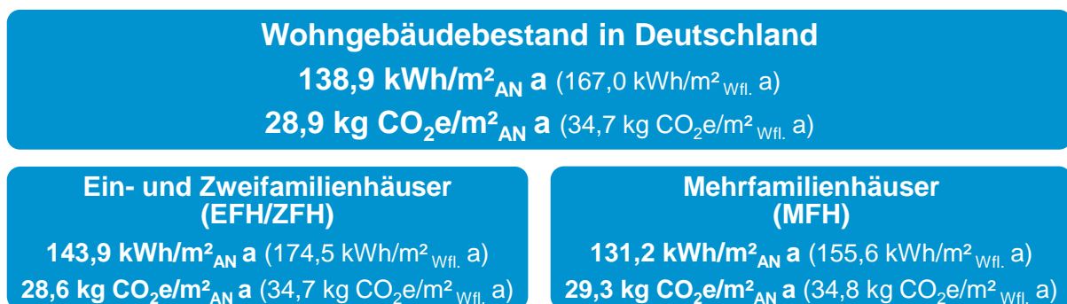
Abbildung 6: Tabellenschema unter Nennung der Kennwerte des Endenergieverbrauchs und der CO 2 e-Emissionen (verbrauchsbasiert) für den Wohngebäudebestand in Deutschland und der damit verbundenen Teilergebnisse für die untersuchten Gebäudetypen (klimabereinigter Energieverbrauch an Endenergie für Heizung und Warmwasserbereitung inkl. Hilfsenergie; Grundlage: Eigene Datenerhebung/-analysen im Bottom-up-Verfahren nach Verursacherprinzip), Bezug: Bestand an Wohngebäuden am 31.12.2020 (ohne Wohnheime)
