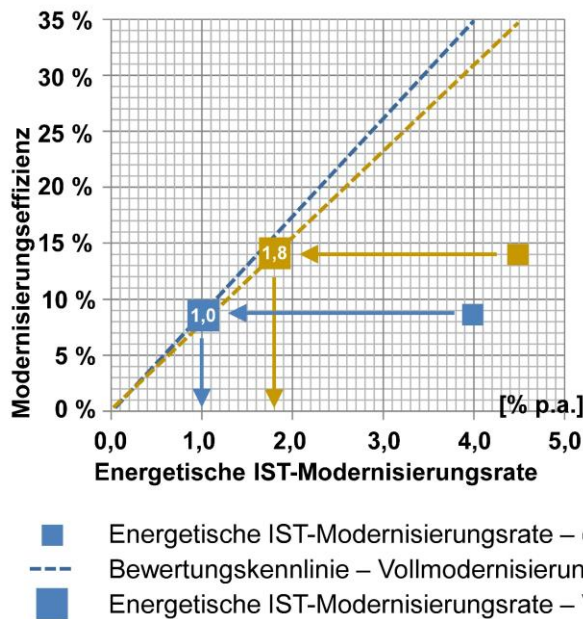
Abbildung 26: Effizienz-Quoten-Diagramm mit Darstellung der heute (Bezug: Bestand an Wohngebäuden am 31.12.2020 (ohne Wohnheime)) im deutschen Wohngebäudebestand vorhandenen Verhältnisse (Blau) und eines fiktiven Erläuterungsbeispiels (Gelb)
