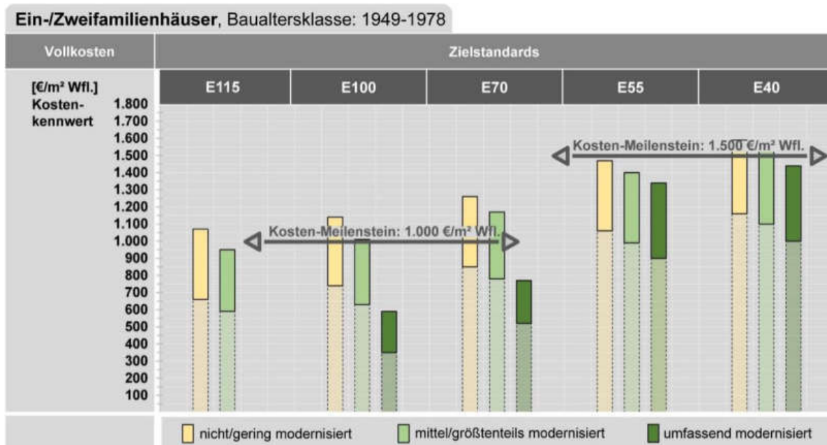
Abbildung 33: Darstellung der unterschiedlichen Kostenniveaus (Vollkosten) der energetischen Gebäudemoder- nisierung in Abhängigkeit zum Ausgangszustand und zum angestrebten energetischen Zielstandards, Ein-/ Zwei- familienhäuser der Baualtersklasse 1949-1978; Grundlage: Auswertung durchgeführter und abgerechneter Mo- dernisierungsvorhaben in Deutschland; Kostenstand: 3. Quartal 2021; Angaben in Form von spezifischen Kos- tenspannen in Euro je Quadratmeter Wohnfläche, inkl. Mehrwertsteuer (Bruttokosten)
