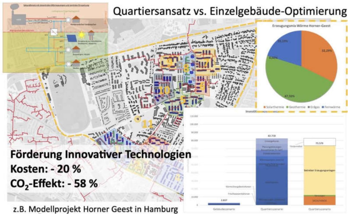
Abbildung 38: Quartierskonzept Horner Geest 149 – Vergleich zweier konkreter Szenarien zur Umsetzung: Einem Gebäudeszenario, das auf die Optimierung der einzelnen Gebäude setzt (Effizienzhaus-Strategie) und der Versorgung durch die Hamburger Fernwärme einschließlich deren Dekarbonisierungspfad setzt, versus eines Quartierszenarios, das bei der Modernisierung (im Mittel) auf ein Effizienzhaus 115, beim Neubau auf einen Standard
