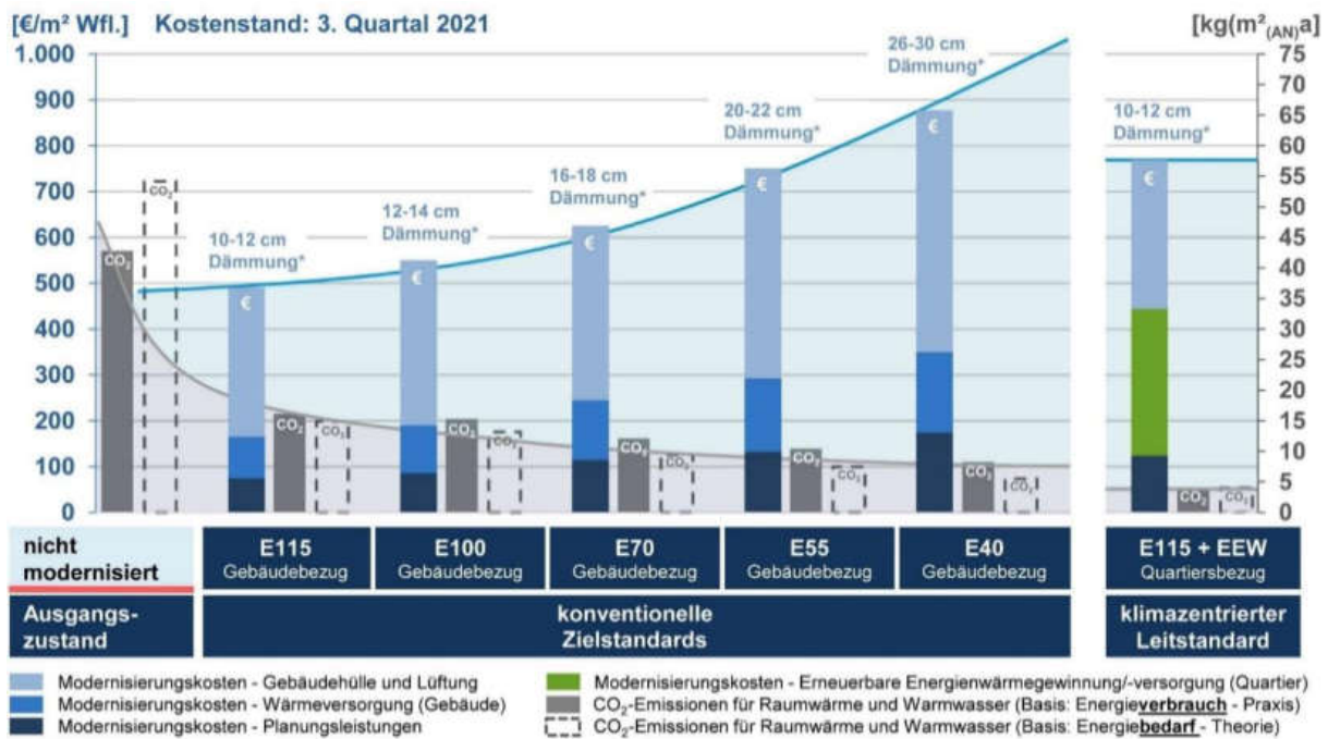
Abbildung 36: Der Zusammenhang von Modernisierungskosten bei Wohngebäuden und CO 2 -Emissionen zeigt deutlich, dass auch im Gebäudebestand eine Überoptimierung des Einzelgebäudes unter Klimaschutzaspekten wirtschaftlich und technisch nicht sinnvoll ist. Vielmehr muss eine deutlich stärkere wirtschaftliche Hinwendung zu innovativen Lösungen bei der Energieversorgung und der Dekarbonisierung der Energieträger angestrengt werden. Das „Effizienzhaus 115“ in Kombination mit intelligenter, erneuerbarer Energieversorgung ist als mittlerer „klimazentrierter Leitstandard“ die wirtschaftlichste Art die Klimaschutzziele und einen „nahezu klimaneutralen Gebäudebestand“ zu erreichen.
