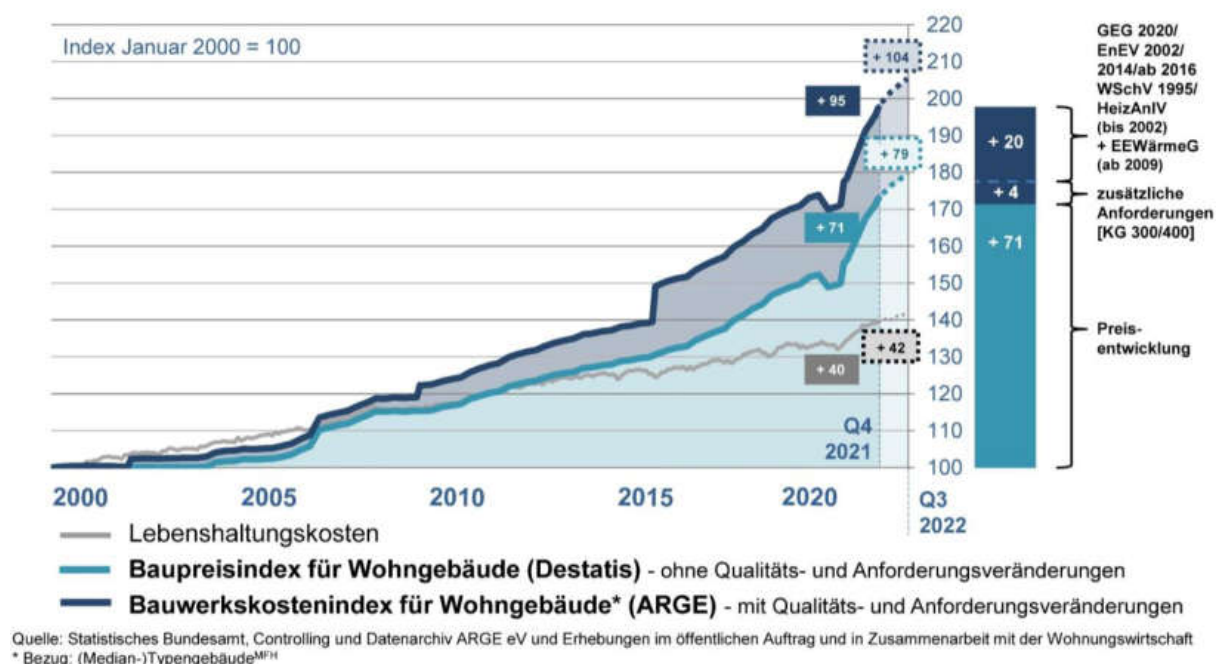
Abbildung 16: Entwicklung der Bauwerkskosten im Wohnungsneubau (Destatis-Preisindex/ARGE-Kostenindex, Bezug: Typengebäude MFH 77 ) unter Berücksichtigung der Mehrwertsteuer im Vergleich zu den allgemeinen Lebenshaltungskosten; Zeitraum: 1. Quartal 2000 bis 4. Quartal 2021 sowie prognostiziert für das 3. Quartal 2022 Quelle: Statistisches Bundesamt, Controlling und Datenarchiv ARGE eV sowie Erhebungen im öffentlichen Auftrag in Zusammenarbeit mit der Wohnungswirtschaft
